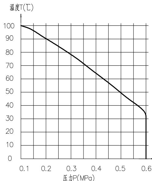
滤室内工作压力P(MPa)与使用温度T(°C)关系曲线图 注:如需高温高压滤板另配制
