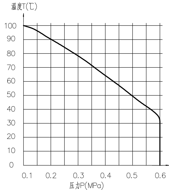
滤室内工作压力P(MPa)与使用温度T(℃)关系曲线图
